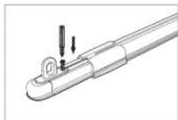
Montează căpăcelele de la capete și strânge șuruburile.
