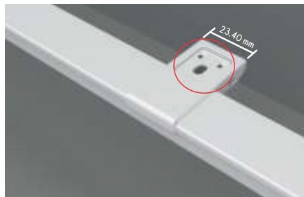
Prindere exterioară (pentru șina superioară) Greutate susținută/prindere - 15 kg Grosime prindere: 1.0 mm \pm 0.02 mm
