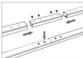
Conectează șina principală cu conectorul din aluminu, aliniază găurile pentru șuruburi și strânge șuruburile.
