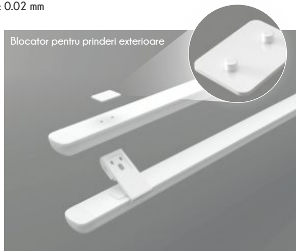
Funcție clips: previne mișcarea șinei atunci când perdelele sau draperiile sunt trase cu forță după instalare.
