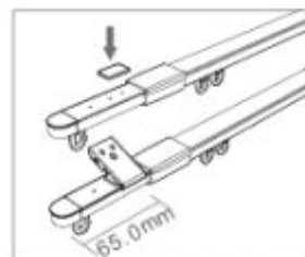
Pe șina secundară trebuie montat un blocator pentru prinderi, iar apoi fixat un clips.
