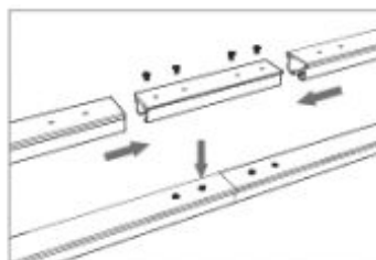
Conectează șina principală cu conectorul din aluminiu, aliniază găurile pentru șuruburi și strânge șuruburile.
