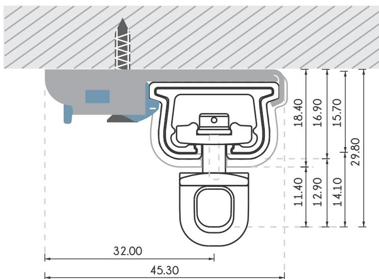
Prindere exterioară (pentru șina superioară) Greutate susținută/prindere - 15 kg Grosime prindere: 1.0 mm \pm 0.02 mm
