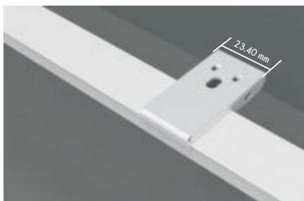
Prindere interioară (pentru șina interioară) Greutate susținută/prindere - 15 kg Grosime prindere: 1.0 mm \pm 0.02 mm
