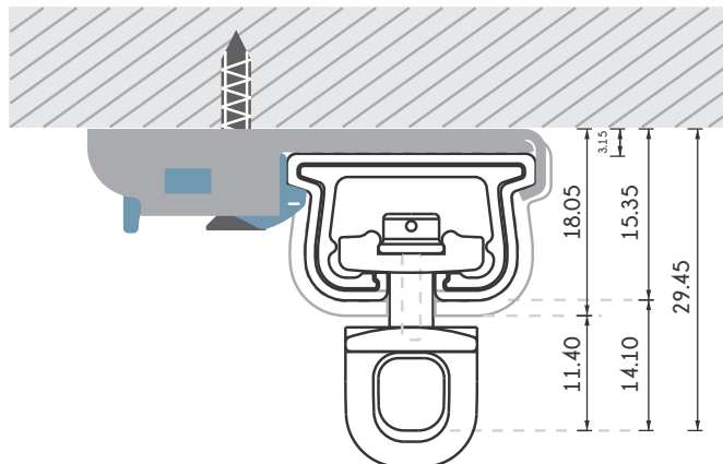
Înălțime totală șină și accesorii
