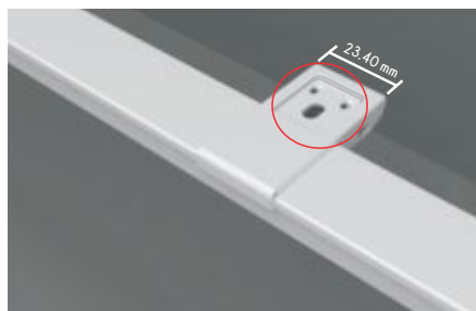
Prindere exterioară (pentru șina superioară) Greutate susținută/prindere - 15 kg Grosime prindere: 1.0 mm \pm 0.02 mm
