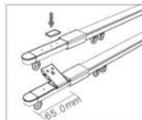
Pe șina secundară trebuie montat un blocator pentru prindere, iar apoi fixat un clips.
